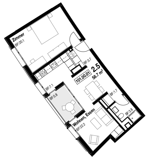
Seminarstr. 101, 1:200
