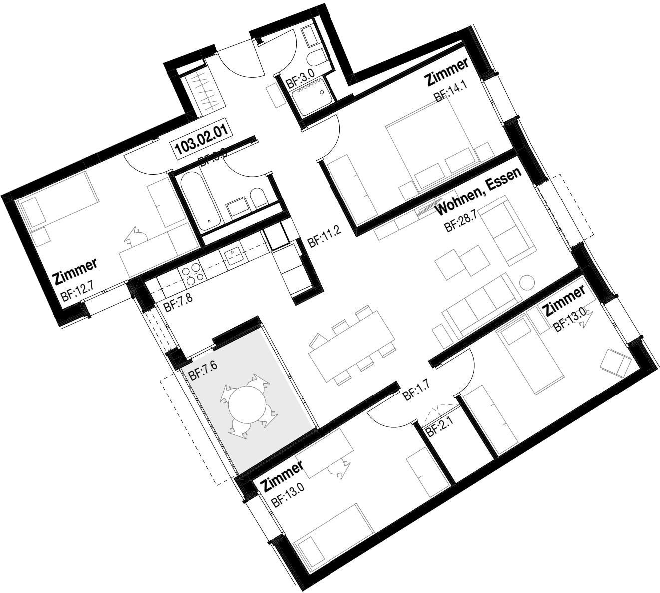
Seminarstr. 103, 1:100, Möblierungsvariante
