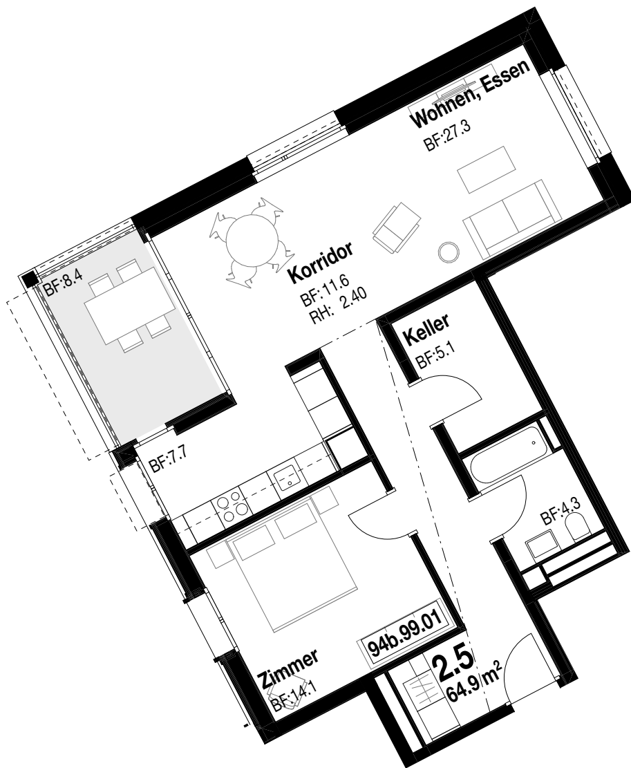
Rötelstr. 94b, 1:100, Möblierungsvariante
