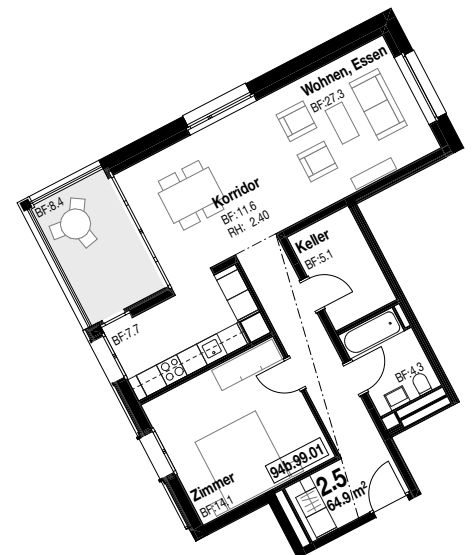
Rötelstr. 94b, 1:200
