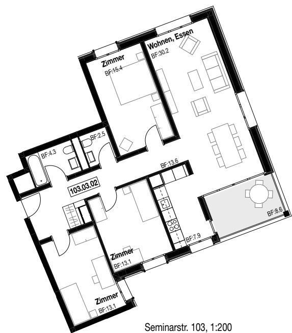
Seminarstr. 103, 1:200
