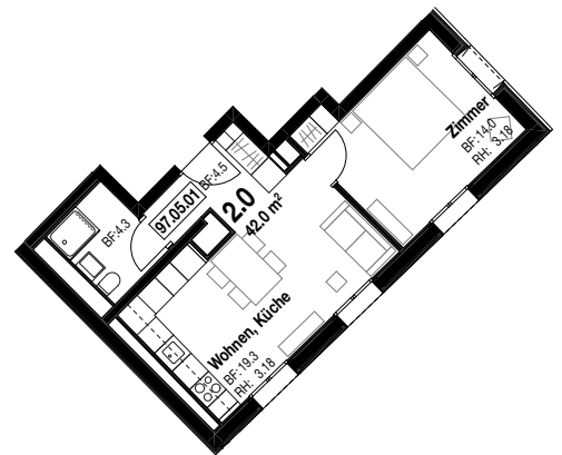
Seminarstr. 97, 1:200
