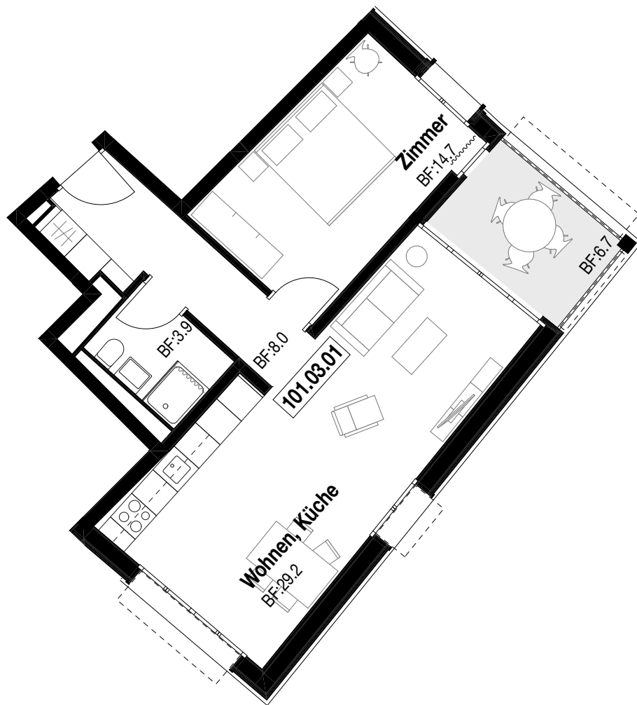
Seminarstr. 101, 1:100, Möblierungsvariante
