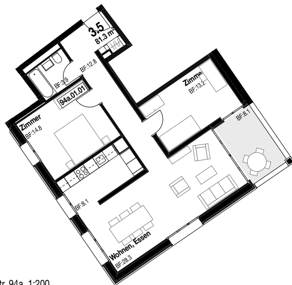
Rötelstr. 94a, 1:200
