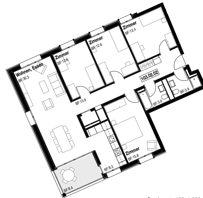
Seminarstr. 103, 1:200
