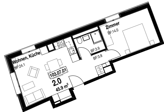
Seminarstr. 103, 1:200
