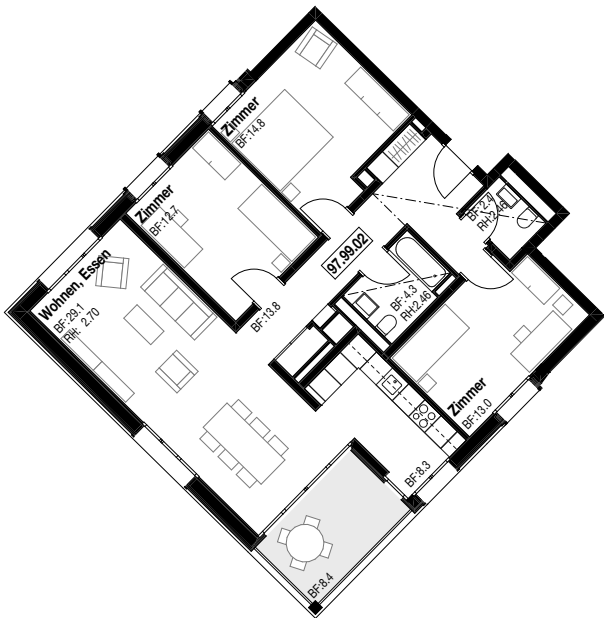
Seminarstr. 97, 1:200
