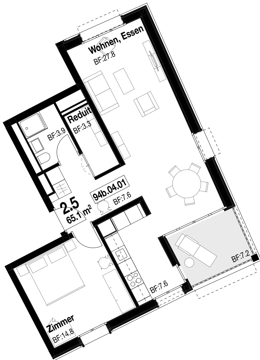
Rötelstr. 94b, 1:100, Möblierungsvariante
