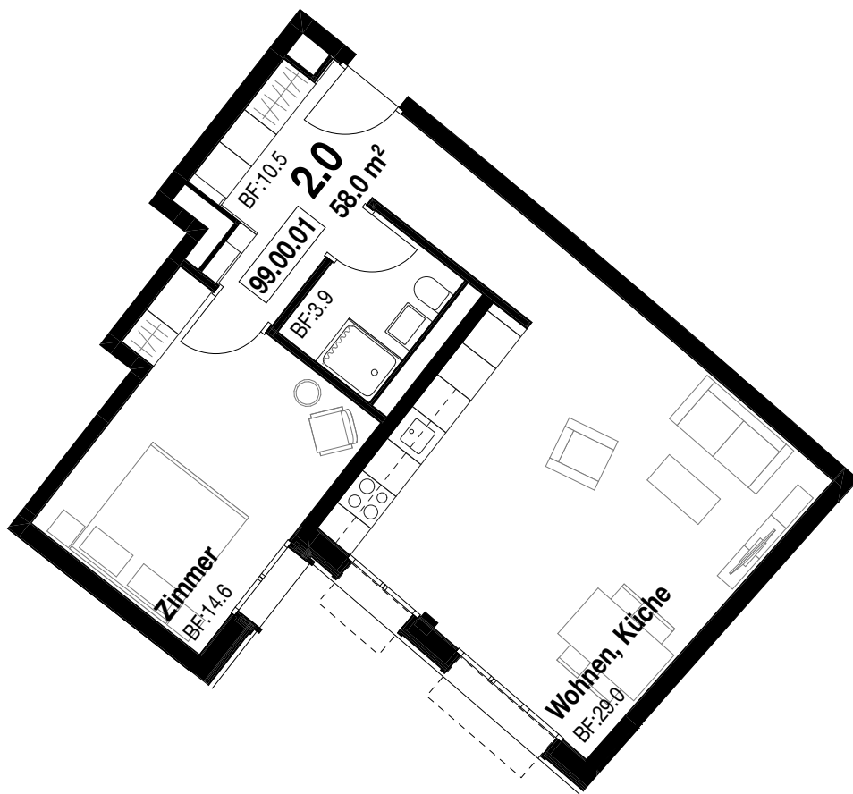
Seminarstr. 99, 1:100, Möblierungsvariante
