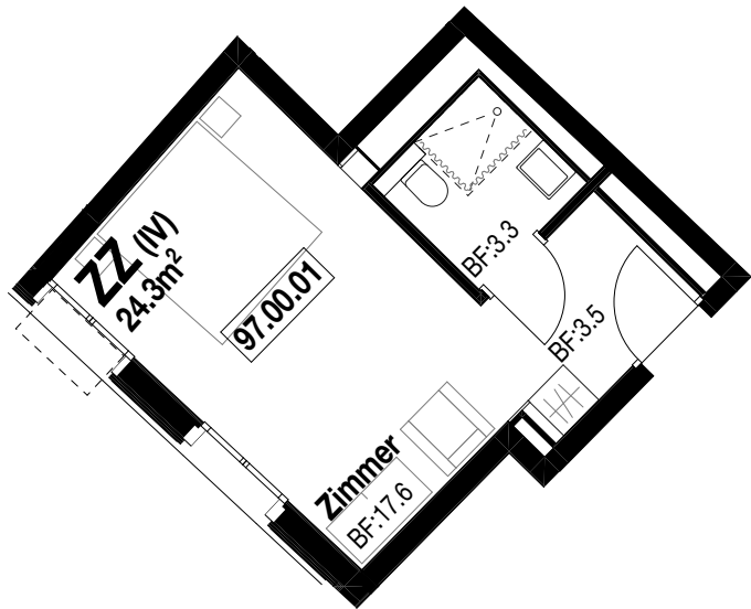
Seminarstr. 97, 1:100
