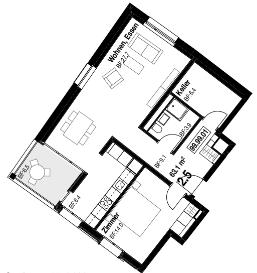
Seminarstr. 99, 1:200
