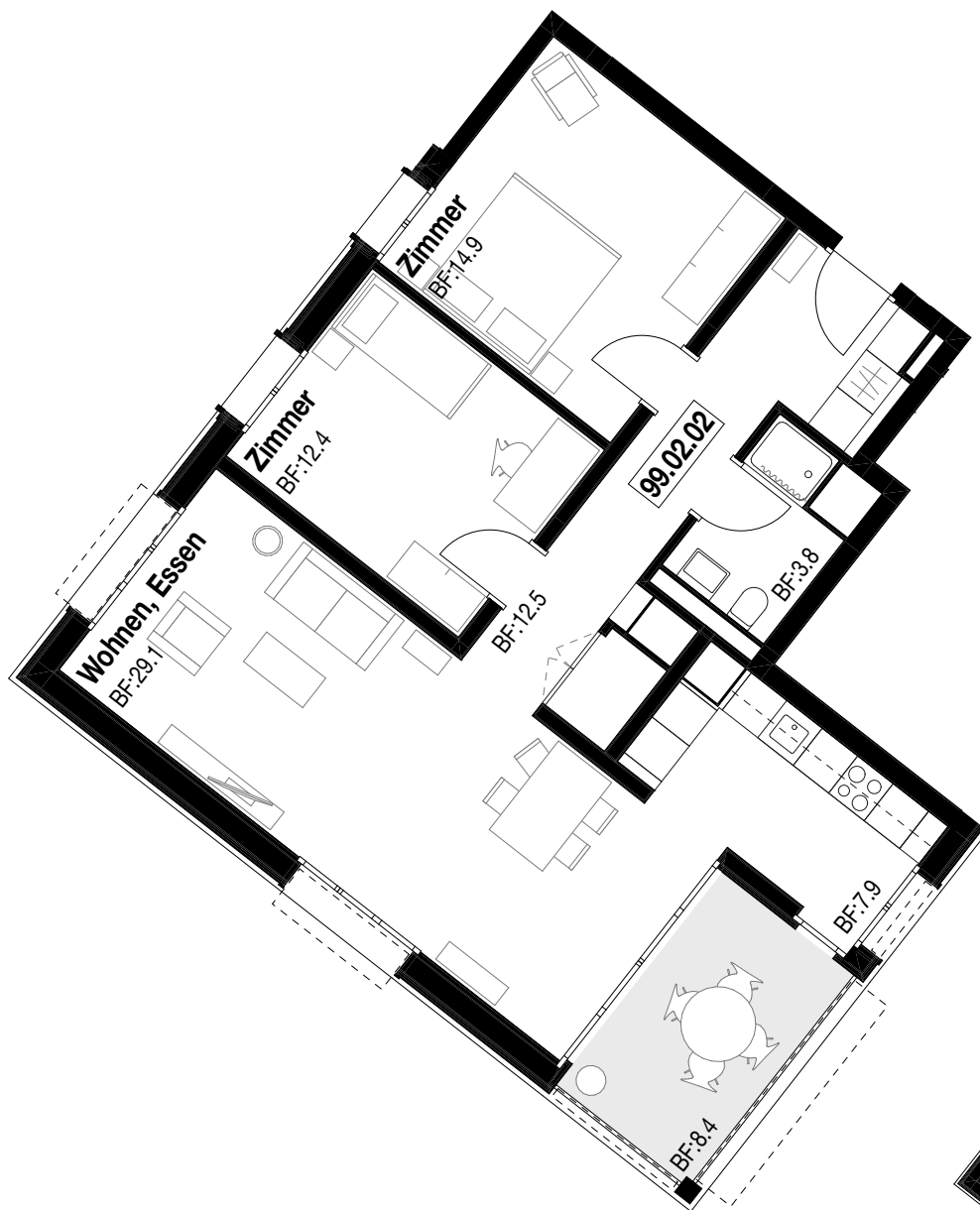
Seminarstr. 99, 1:100, Möblierungsvariante
