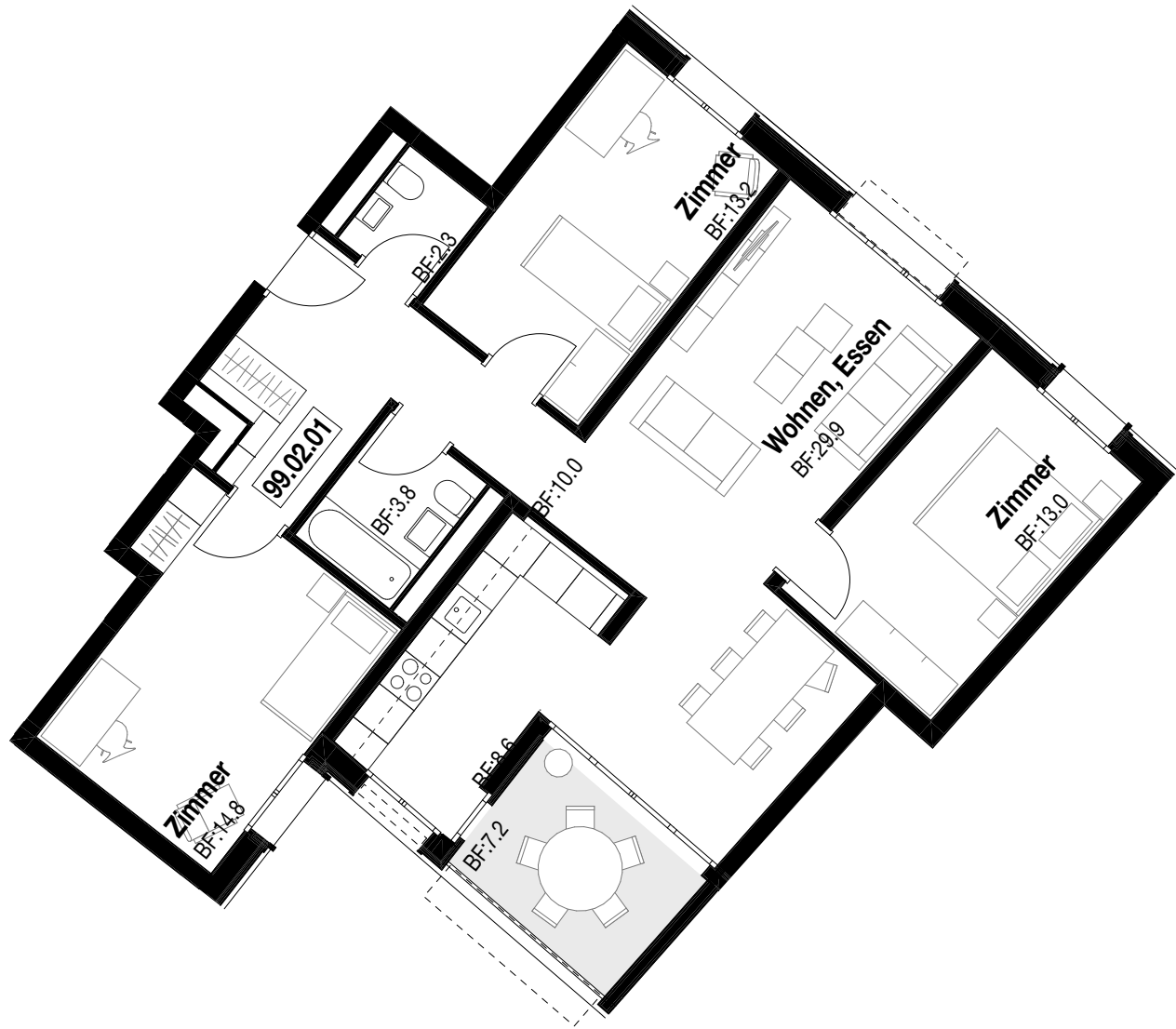
Seminarstr. 99, 1:100, Möblierungsvariante
