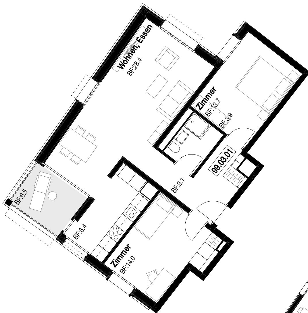
Seminarstr. 99, 1:100, Möblierungsvariante
