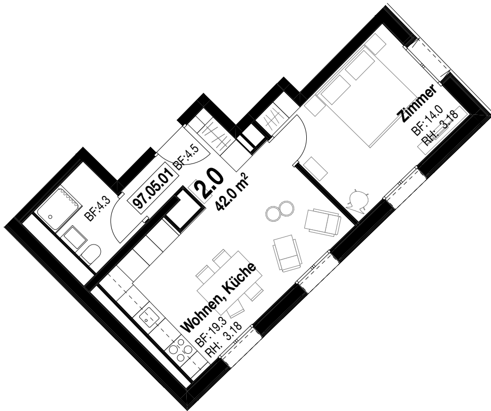
Seminarstr. 97, 1:100, Möblierungsvariante
