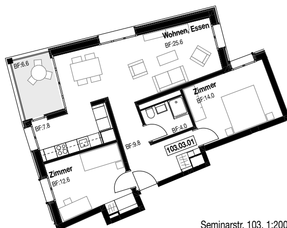
Seminarstr. 103, 1:200
